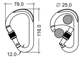
SCREW SLEEVE #786MA0NNKK
